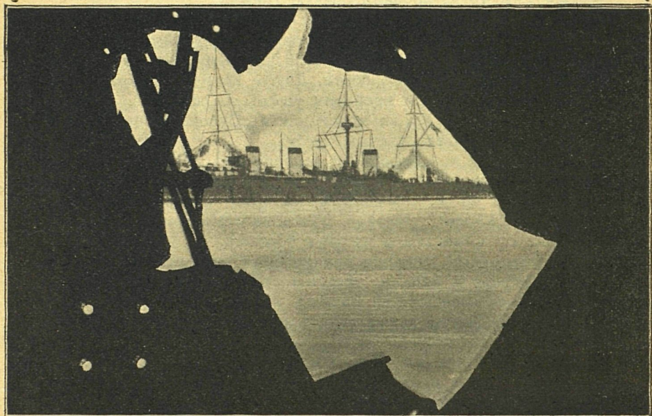
„Олегъ“ послѣ боя. Самая большая пробоина въ корпусѣ, черезъ которую видѣнъ крейсеръ „Жемчугъ“.
