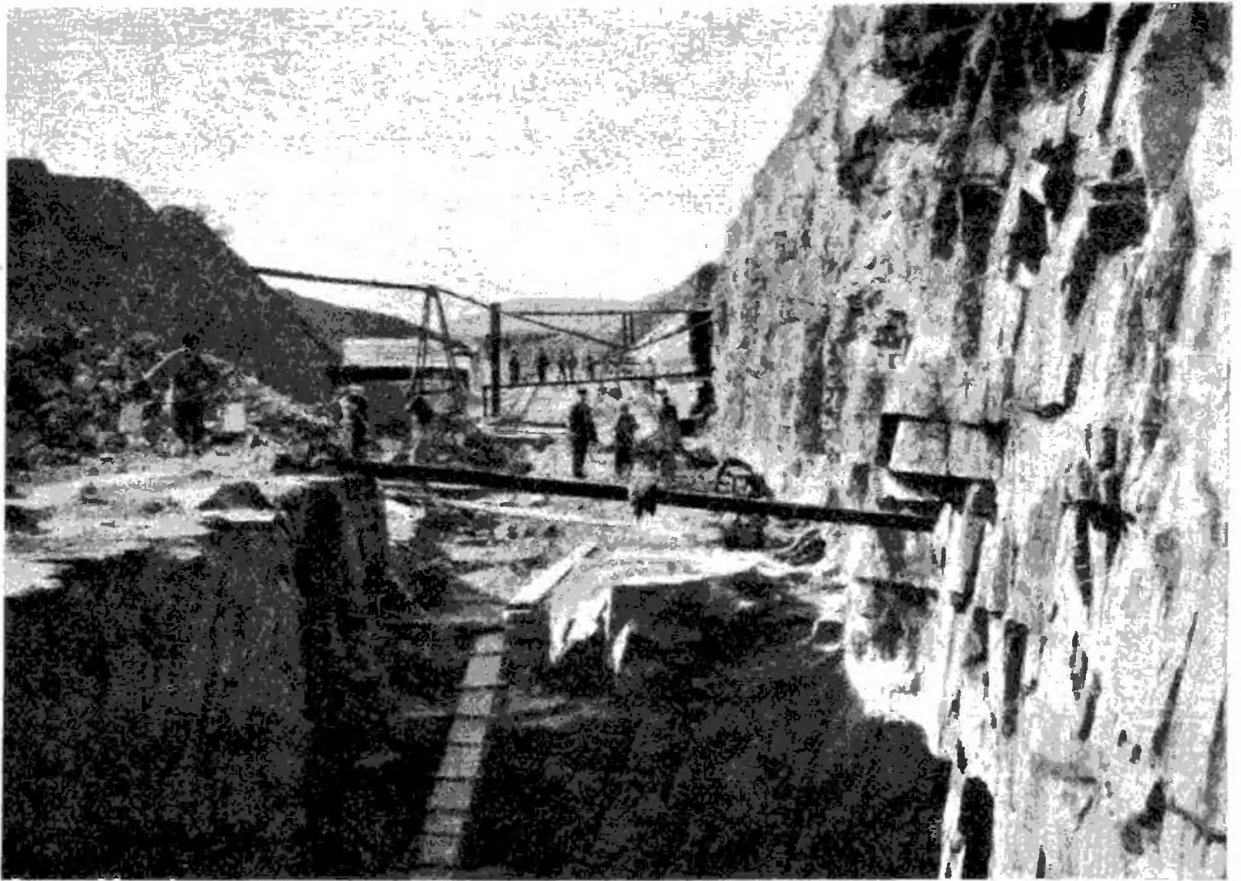
Горжевой ровъ укрѣпленія № 4 во время постройки.
