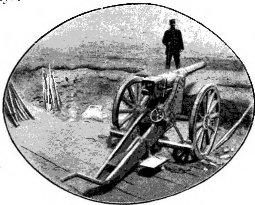
87 м.м. орудіе на бат. № 4. (Снято японцами послѣ боя).
