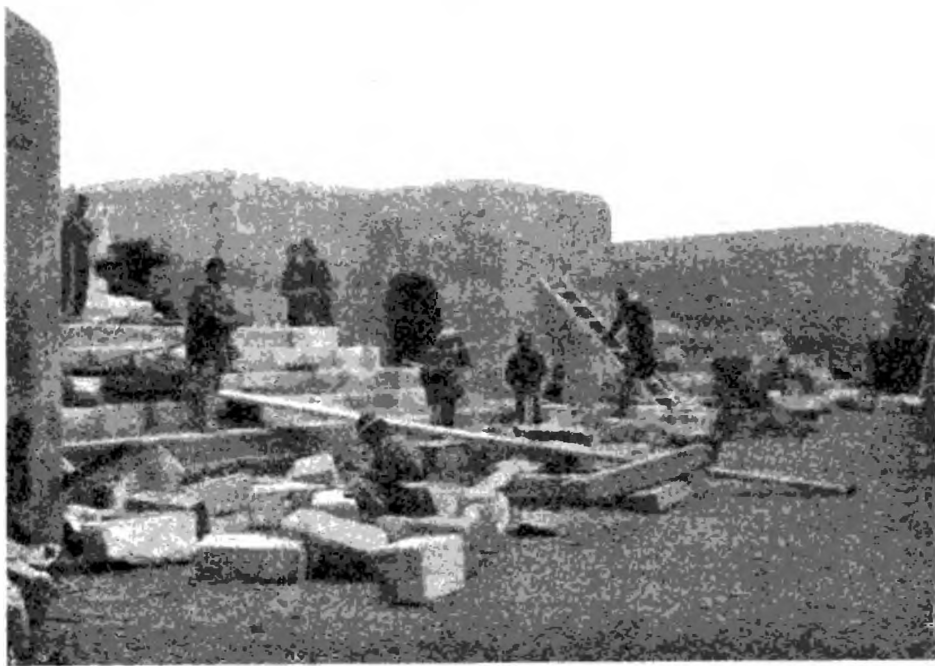
Постройка гнѣздъ для 75 м/м орудій на флангъ бат. № 15.
